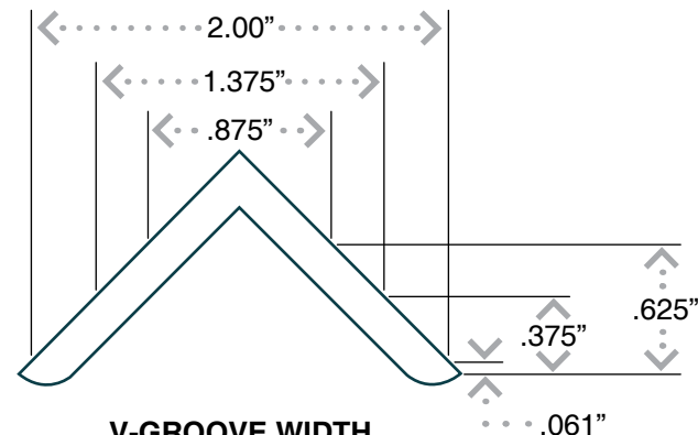
V-GROOVE WIDTH
