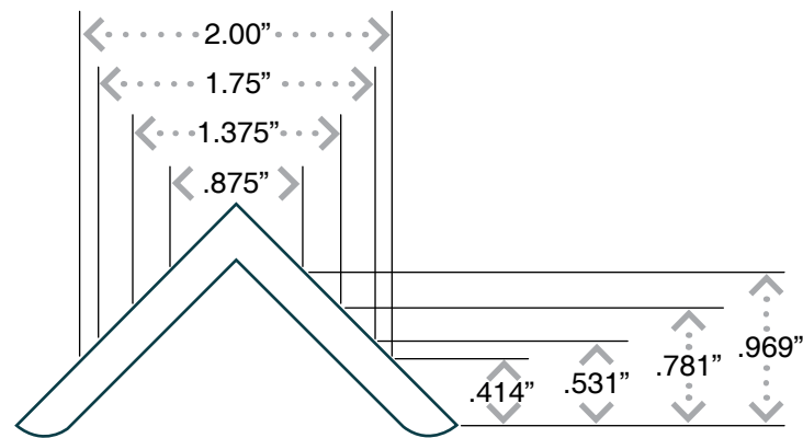
V-GROOVE WIDTH
